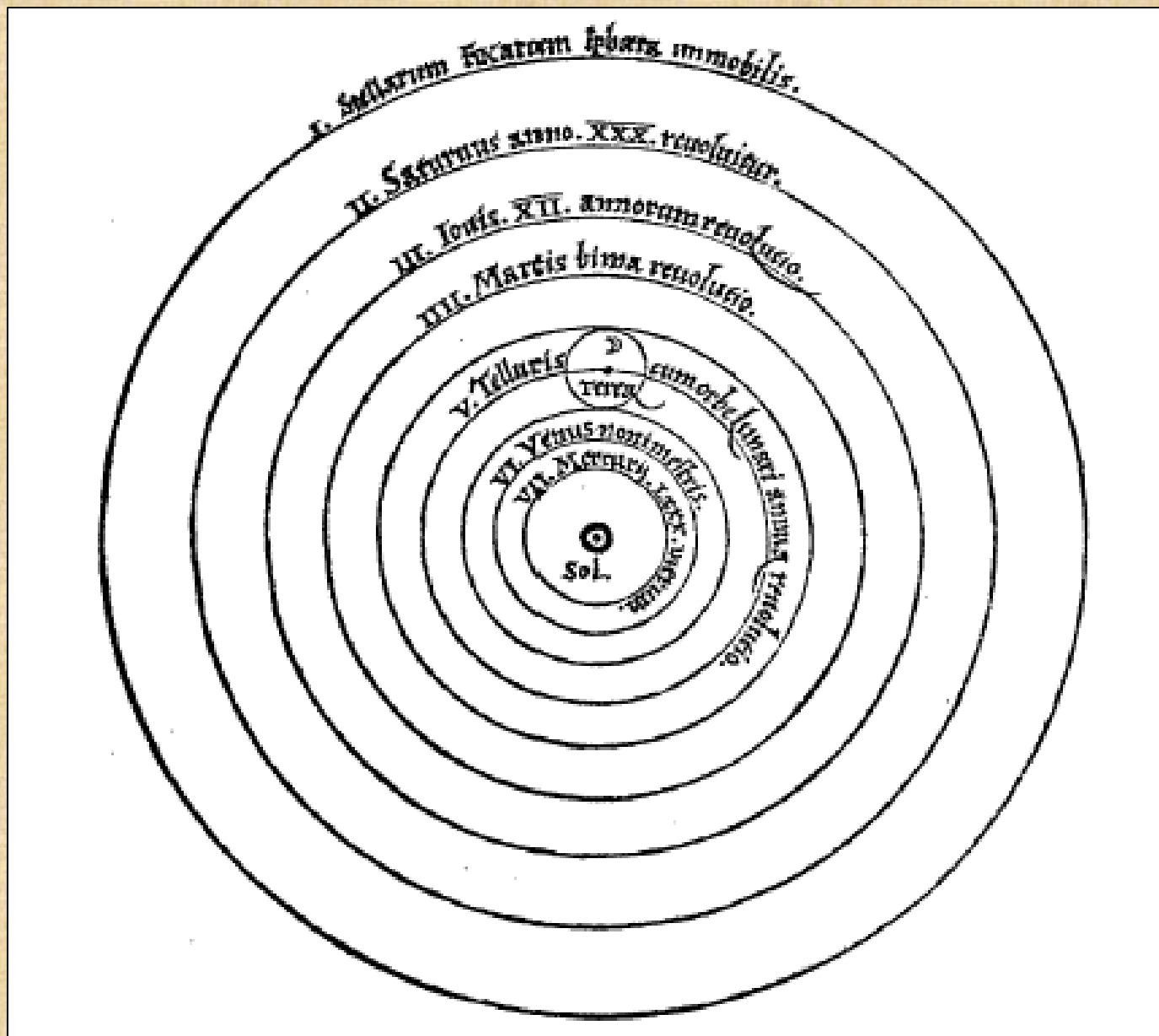
Sistema heliocéntrico de Copérnico simplificado
